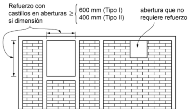
Figura 0.3 Reforzo en el perímetro de aberturas
